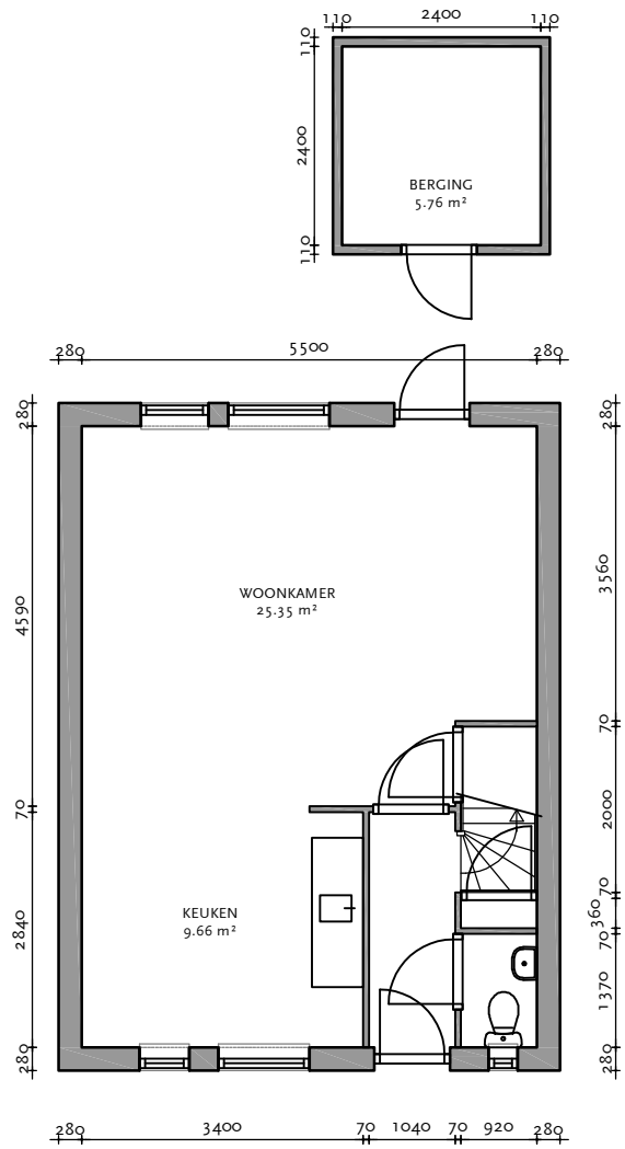
Begane grond
