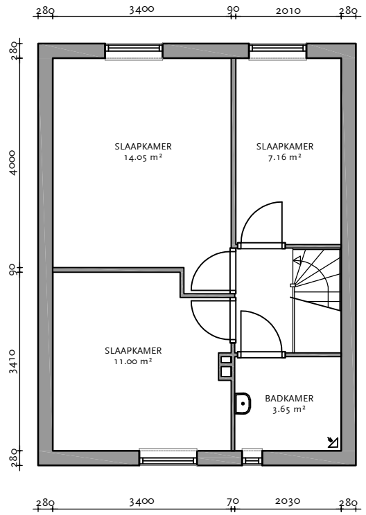
Verdieping
